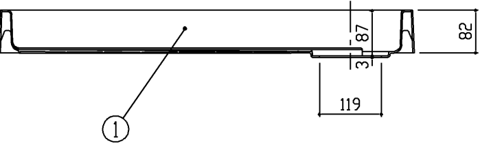
断面A-A
